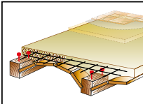
Bigueta de fusta i revoltons
