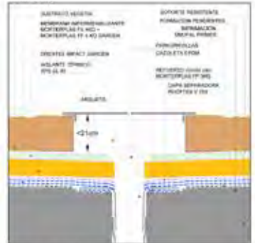
Junta dilatación
